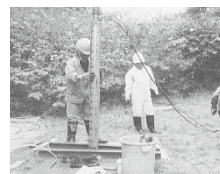
温泉の井戸に水中ポンプを設置している様子
