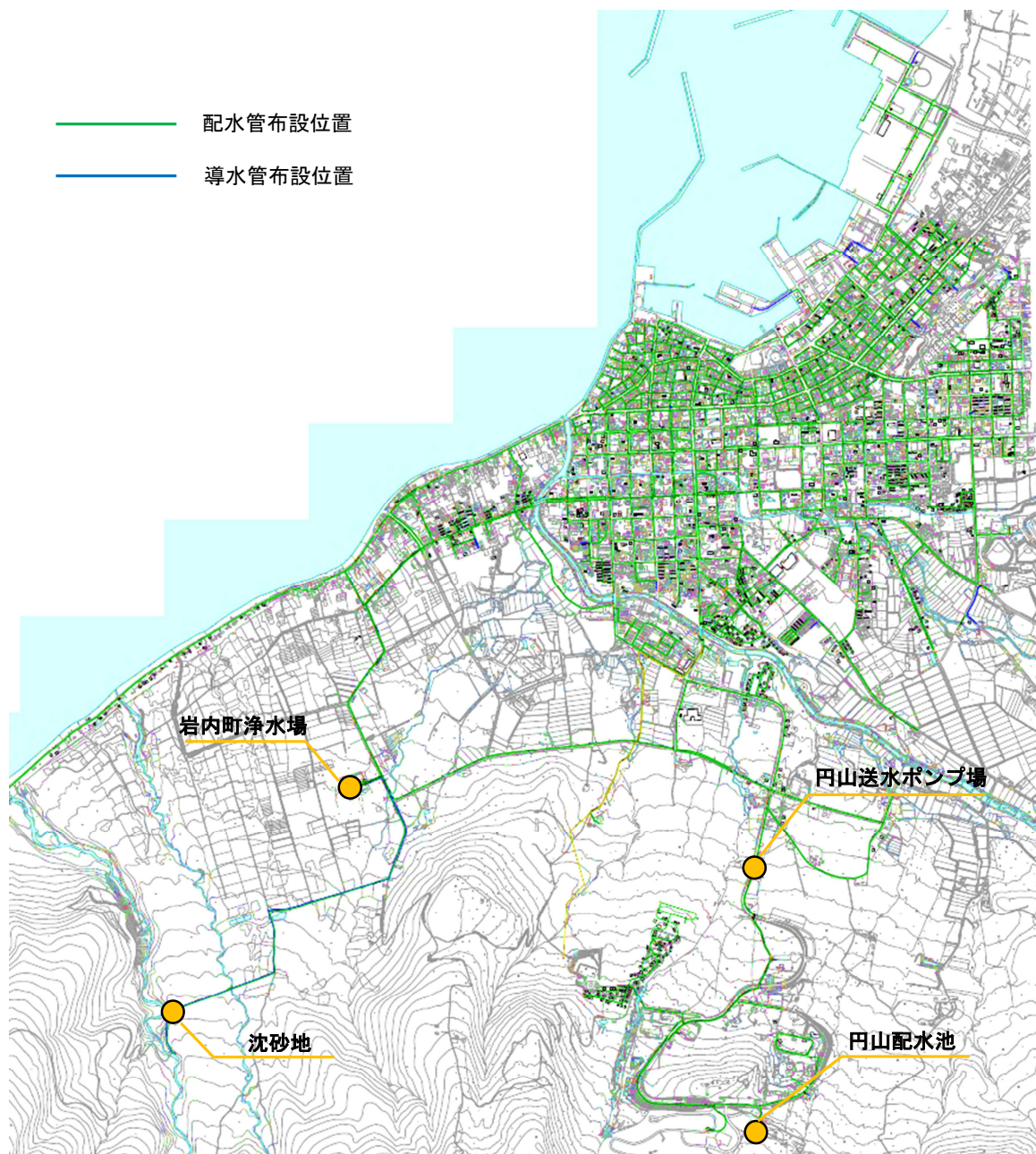
図 岩内町浄水場・導水管および配水管布設位置図
