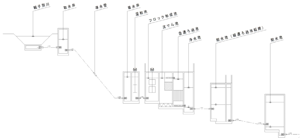
図 雷電地区水道施設フロー
