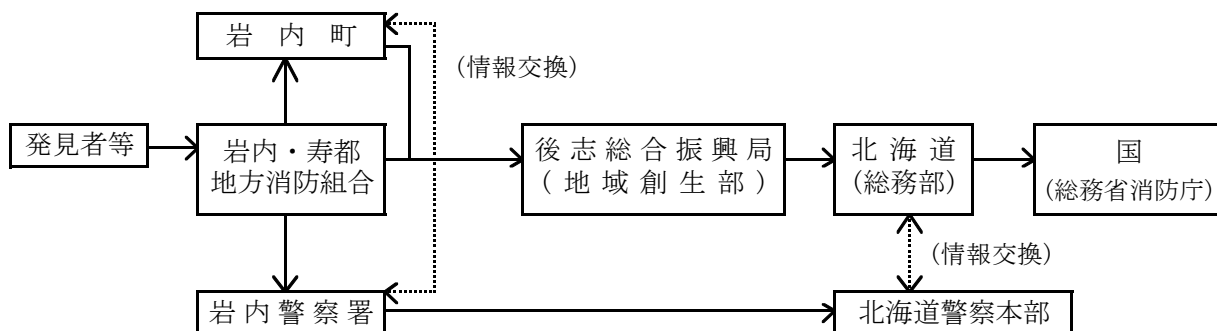
別記 情報通信連絡系統図
